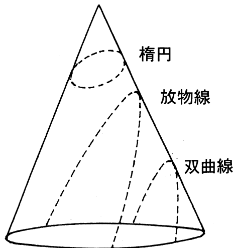
図2 円錐曲線
