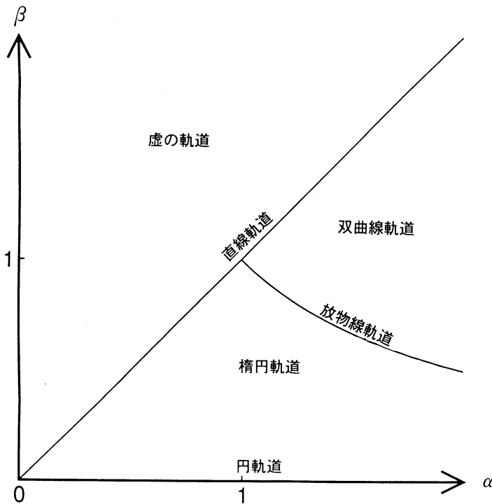
図3 パラメーター \alpha, \beta と軌道の形
